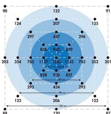
SLIMSUNPRO240W@30cm PPFD = 1260
