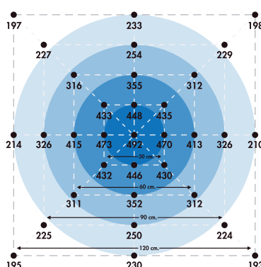
SLIMSUNPRO240W@60cm PPFD = 492
